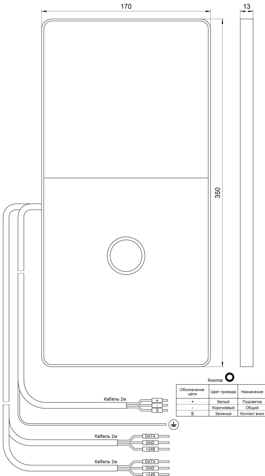
Рис.1 Внешний вид, габаритные и установочные размеры Вызывного поста МАЛАХИТ НШЕК.468381.127
